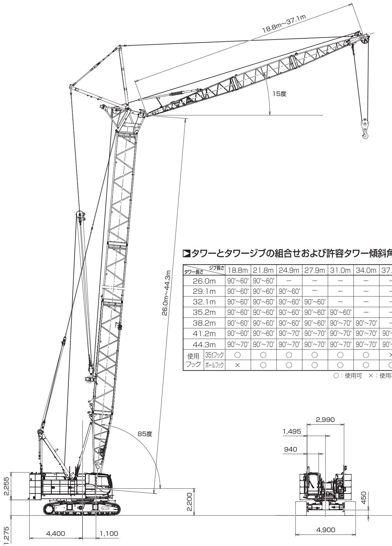
全体図(単位：mm)
